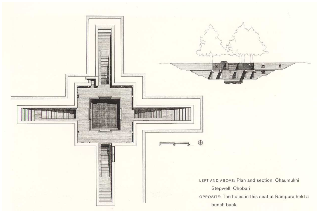
2. חתך ותרשים ממעל של באר Chamukhi ב- Rampura שבסאורשטרה. מתוך: Livingston, עמ' 50.
