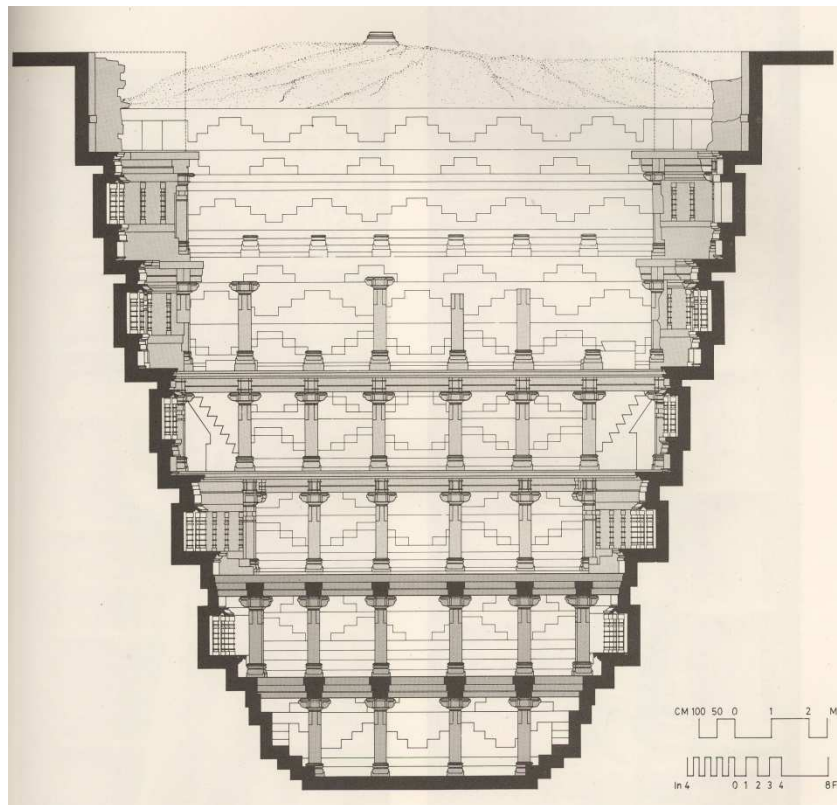
5. באר המדרגות בפטאן. חתך רוחב במבט מזרחה. מתוך: Mankodi, עמ' 193.
