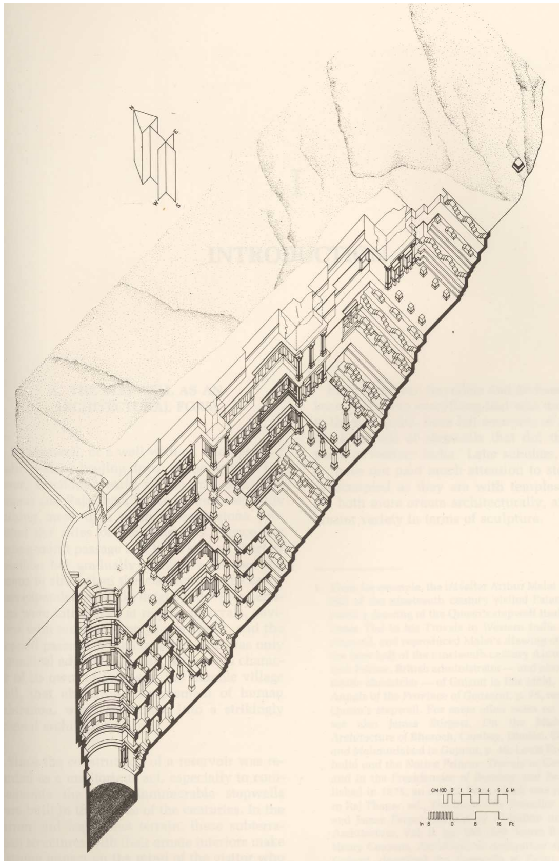
1. באר המדרגות בפטאן. חתך במבט על. מתוך: Mankodi.
