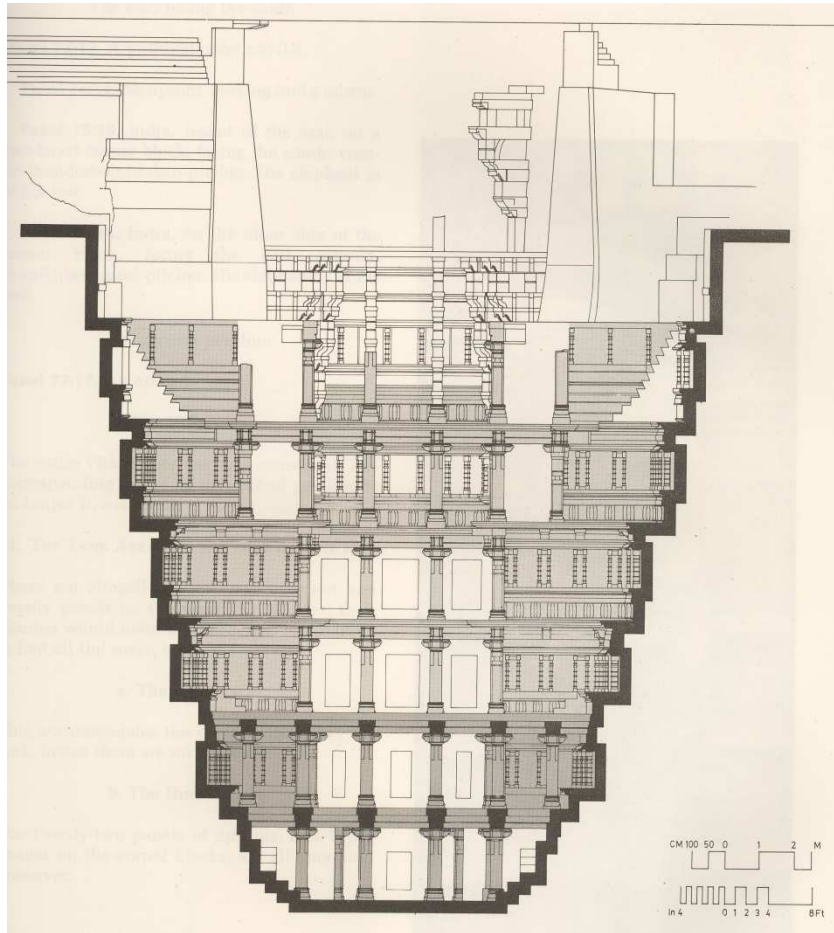
4. באר המדרגות בפטאן. חתך רוחב במבט מערבה. מתוך: Mankodi, עמ' 185.
