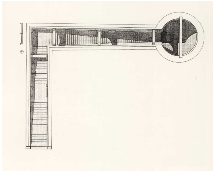
1. תרשים הבאר ב- Dhank, סאורשטרה. מתוך: Livingston, עמ' 24.
